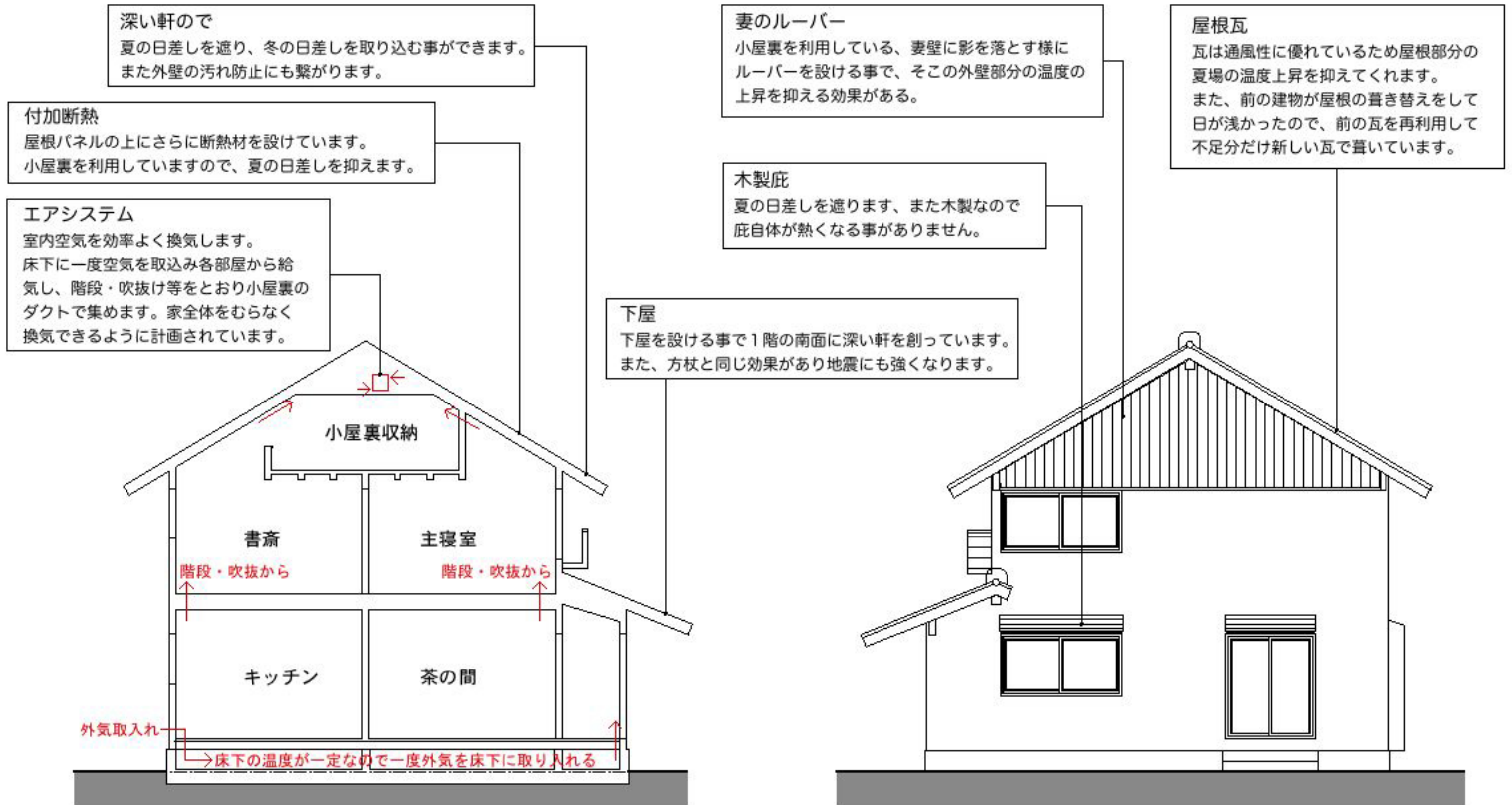
断面図
